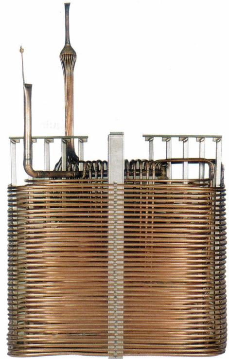
RCU 10 Evaporator.
