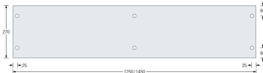
G15-1200G / 1200-Oak / 1400G / 1400-Oak Plan View:
