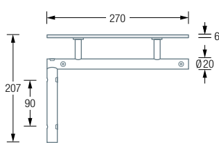
G15-1200G / 1200-Oak / 1400G / 1400-Oak Plan View:
